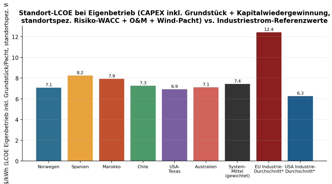
Abb. 6: Validierter Standort-LCOE bei Eigeninvestition (CAPEX-Annuität inkl. Grundstückskosten bei standortspezifischem Risiko-WACC von 5,5–9,5 % über 20 Jahre + 2 % O&M + Wind-Pachtkosten) im Vergleich zu allgemeinen Industriestrom-Referenzwerten für die USA und die EU (*IEA, Electricity 2026: EU-Industriestrompreise 2025 im Schnitt rund doppelt so hoch wie in den USA und ca. 50 % höher als in China).
