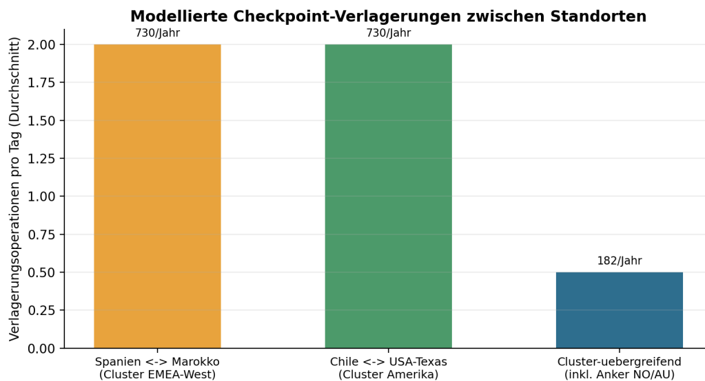
Abb. 5: Modellierter Verlagerungsoperationen pro Tag und Jahr, aufgeschlüsselt nach Cluster-intern (häufig, kurze Distanz, private Glasfaser) und cluster-übergreifend (selten, lange Distanz, öffentliche/gemietete Backbone-Kapazität).
