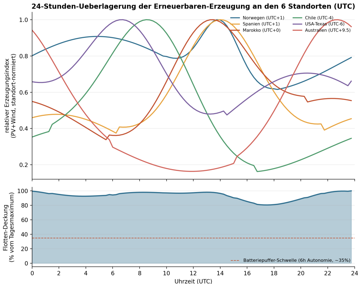
Abb. 3: Oben: modellierter, standort-normierter Erzeugungsindex (PV+Wind) der sechs Standorte über 24 Stunden (UTC). Unten: resultierende Deckung der Gesamtflotte in Prozent des Tagesmaximums; die gestrichelte Linie markiert die Schwelle, ab der die 6-Std.-Batteriepufferung nicht mehr ausreicht und eine Verlagerung ausgelöst wird.
