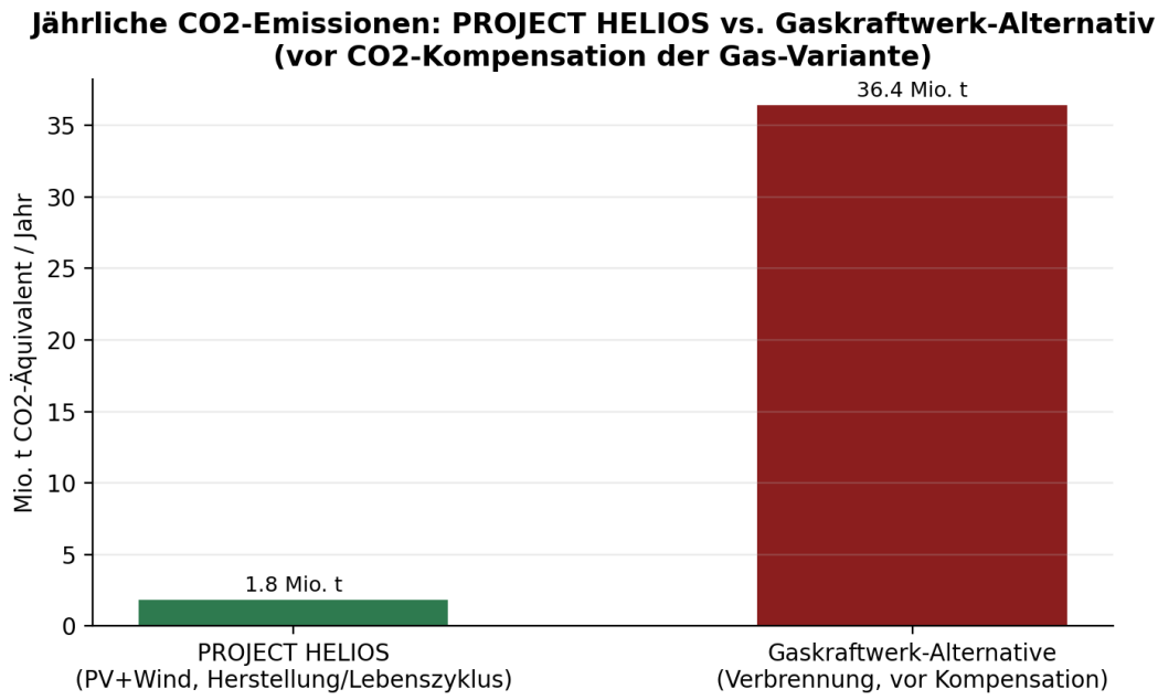
Abb. 9: Jährliche CO2-Emissionen im Vergleich. PROJECT HELIOS verursacht nur Lebenszyklus-/Herstellungsemissionen (Produktion & Errichtung von PV-Modulen, Windturbinen und Batterien, grob mit 20–25 g CO2/kWh über die Lebensdauer amortisiert angenommen), während die Gas-Alternative rund 36,4 Mio. t CO2/Jahr direkt emittiert, die erst nachträglich durch Zertifikate kompensiert werden müssen.
