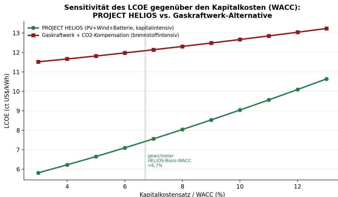
Abb. 7a: Sensitivität des LCOE gegenüber dem Kapitalkostensatz (WACC), im Vergleich zwischen PROJECT HELIOS (kapitalintensiv, \approx 100 % des LCOE ist Kapitalkosten + O&M) und der Gaskraftwerk-Alternative (kapitalleicht, dominiert von laufenden Brennstoff- und CO 2 -Kosten). Über die dargestellte Bandbreite von 3–13 % WACC schwankt der HELIOS-LCOE um rund 4,8 ct$/kWh, der Gas-LCOE dagegen nur um rund 1,5 ct$/kWh.
