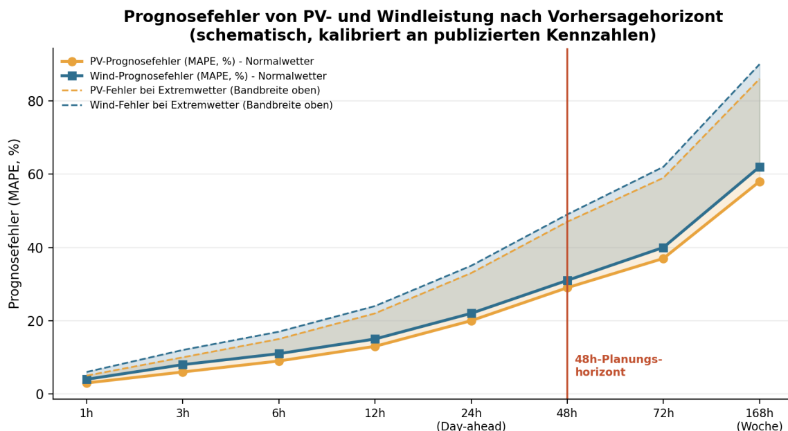
Abb. 7: Schematischer Verlauf des Prognosefehlers (MAPE) für PV- und Windleistung nach Vorhersagehorizont, kalibriert an publizierten Werten für 3h-, Day-ahead- und Wochenvorhersagen ( Exploring the Efficiency of Renewable Energy-based Modular Data Centers at Scale , arXiv 2406.02252). Die gestrichelten oberen Linien zeigen den zusätzlichen Fehleraufschlag bei Extremwetterlagen (eigene Schätzung, siehe 6.2). Die 48h-Marke ist der für dieses Projekt relevante Planungshorizont.
